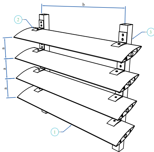
Sơ đồ lắp đặt/ Installation diagram
